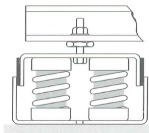
Montage avec mise à niveau
